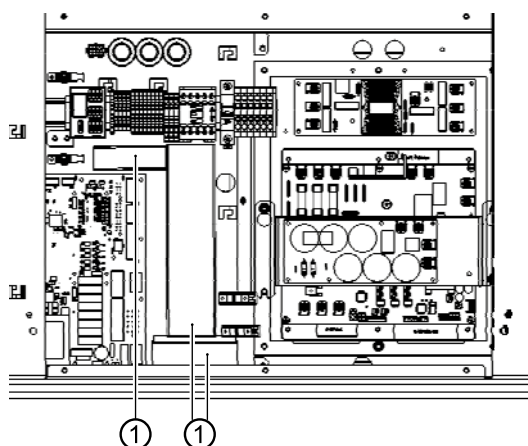
1 Kabelový kanál
